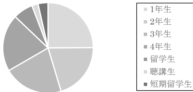
図2 クラス構成
